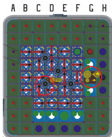
2. ábra: A pneumatikus csőposta rendszer termikus csatornája a „G” oszlopban található.
